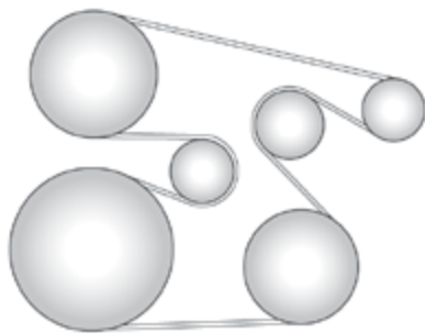
Двигатель 3,6 л V6
