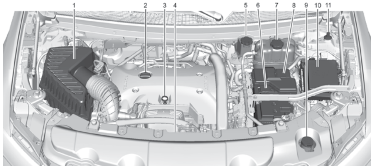
Двигатель 2,0 л L4
