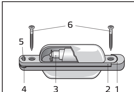
Рис. 62. Фонарь освещения номерного знака
