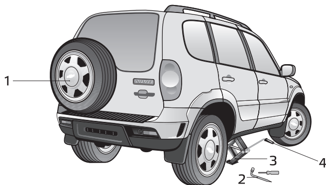
Рис. 56. Подъем автомобиля при замене колёс
