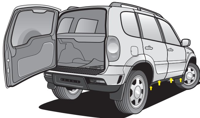
Рис. 65. Дренажные отверстия дверей и порогов
