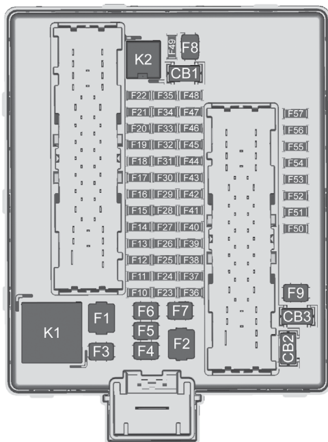
Блок предохранителей, расположенный в багажном отделении
