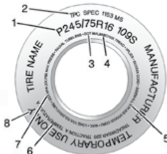
Пример маркировки шин для легкового автомобиля (P-Metric) (шина запасного колеса)
