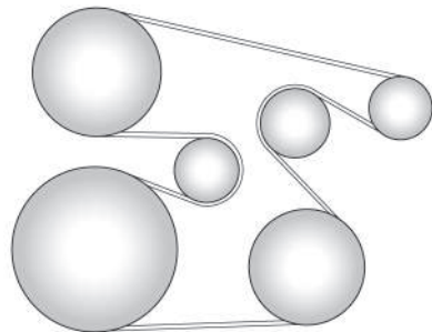
Двигатель 3,6 л V6
