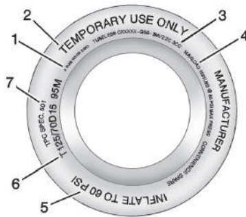
Пример маркировки шины неполноразмерного запасного колеса
