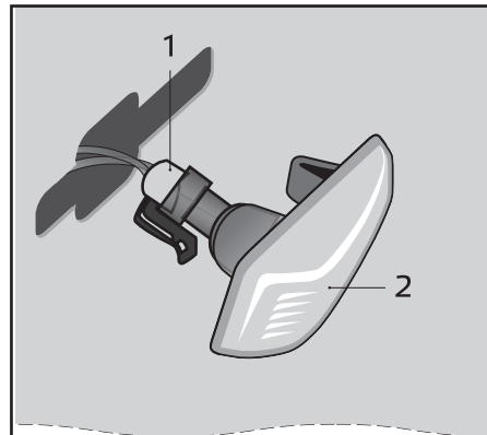
Рис. 71. Боковой указатель поворота
