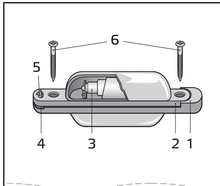
Рис. 70. Фонарь освещения номерного знака
