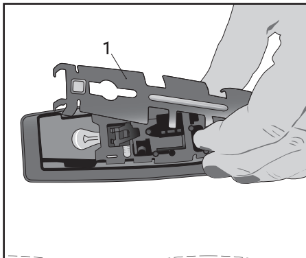
Рис. 69. Задний плафон освещения салона
